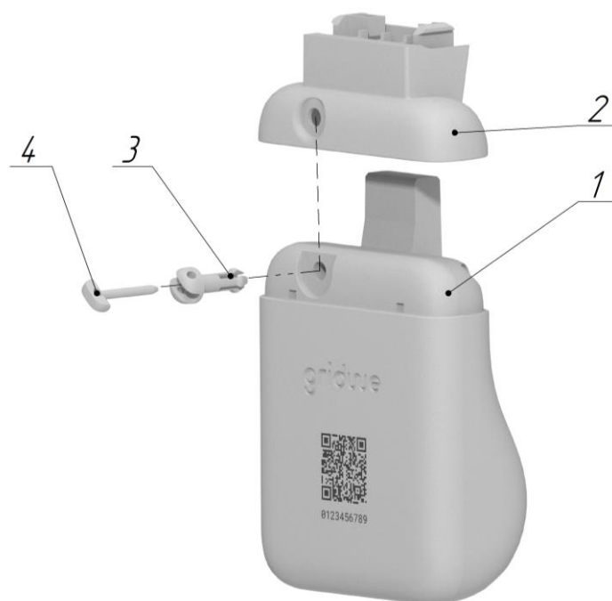
Рисунок 2 - Конструкція модему
