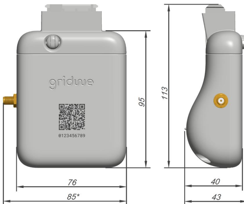
Рисунок 1 - Габаритні розміри модему
