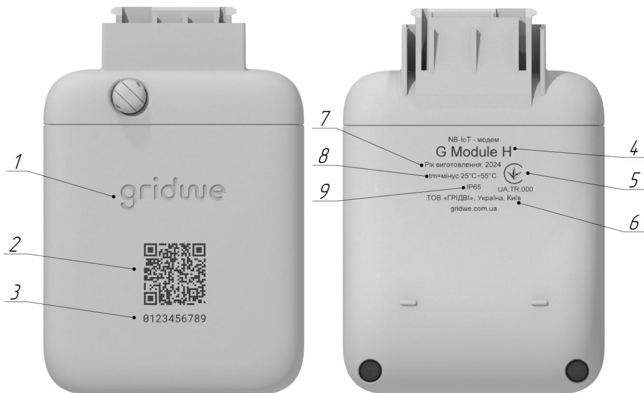
Рисунок 3 - Зразок маркування
