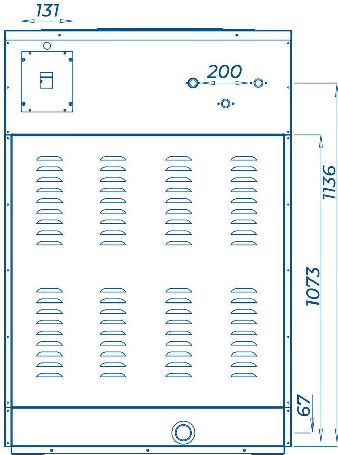
TRASERA
