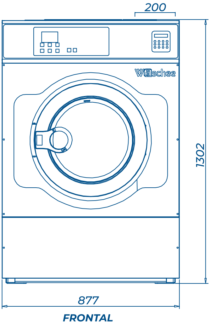
FRONTAL
