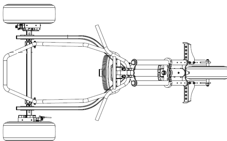
Vue de dessus — architecture du châssis
