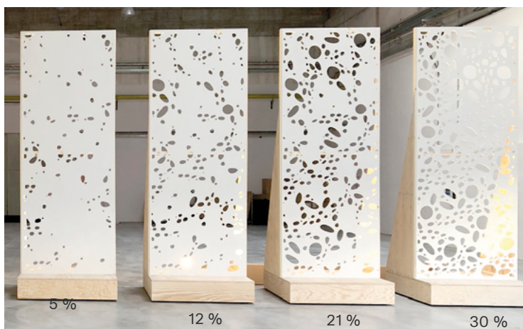
Beispiel elliptische Perforation, variierender Lochanteil
