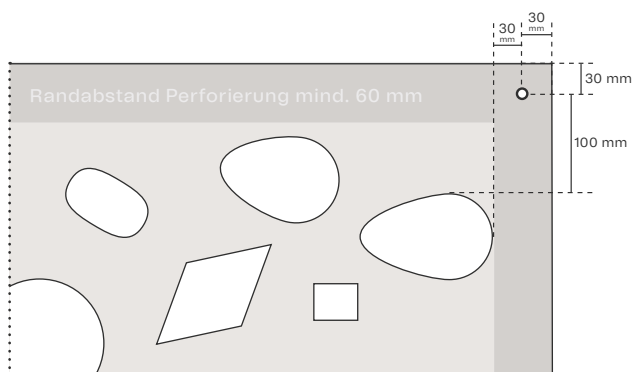
sichtbare Befestigung
