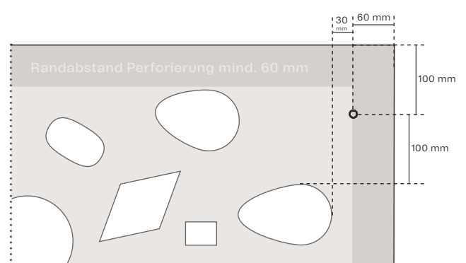
nicht sichtbare Befestigung
