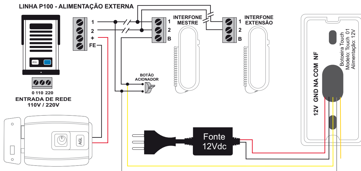
Figura 3 - esquema de ligação com interfone P100
