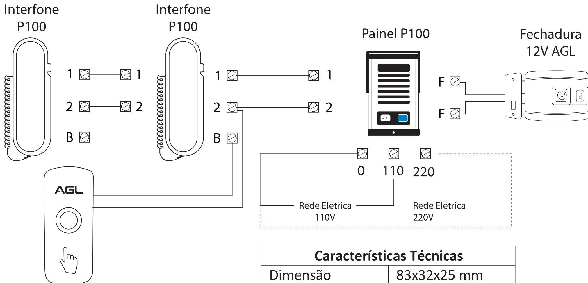
Figura 1 - esquema de ligação com porteiro P100 AGL
