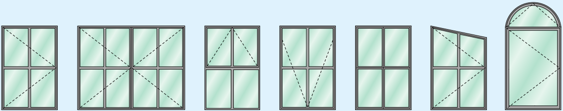
Fenêtre à soufflet et battante
