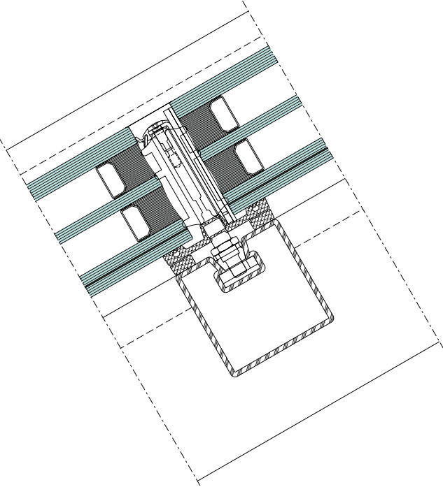
COUPE EN DÉTAIL
