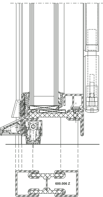
Porte avec seuil zéro
