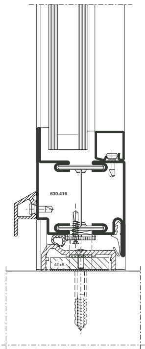
Porte avec seuil sans barrière
