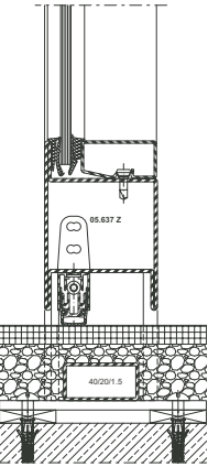
Porte avec seuil zéro
