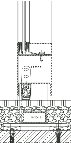
Porte avec seuil zéro
