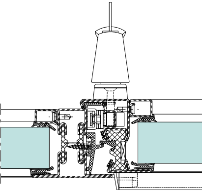
Section de détail Janisol 1
