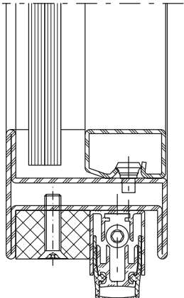
Porte avec seuil zéro
