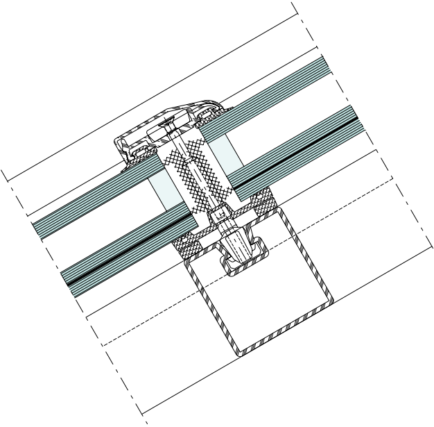
COUPE EN DÉTAIL
