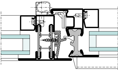
Section de détail Janisol Primo
