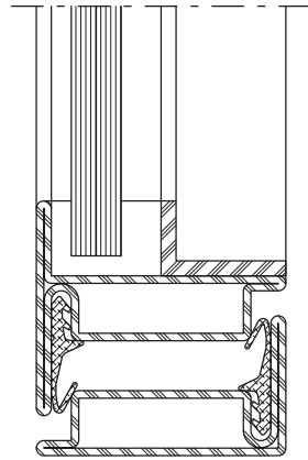
Porte sans barrière
