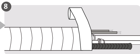
Owiń rury i przewody elektryczne taśmą izolacyjną (nie dotyczy niektórych lokalizacji w USA)
