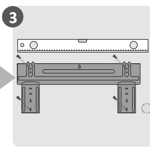
Zamocuj płytę montażową
