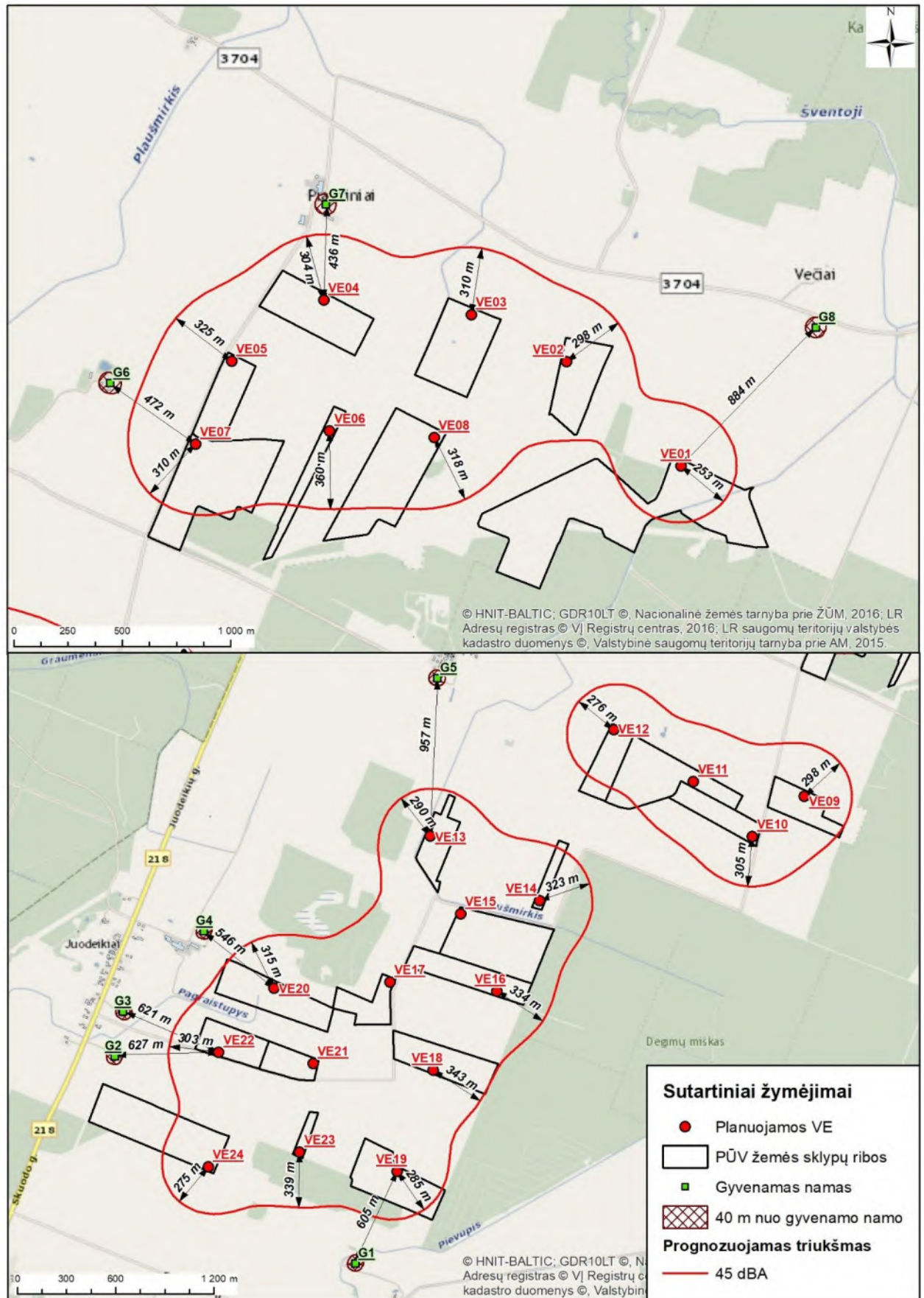
2.11.1a pav. Prognozuojamo PŪV triukšmo lygio izolinijos 40 m atstumo nuo artimiausių gyvenamųjų pastatų atžvilgiu.
