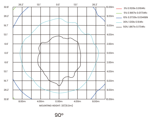
Iso-illuminance Diagram (Iso-lux)
