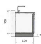
Schnitt M 1:25
