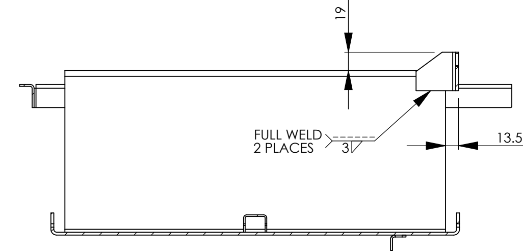
SECTION A-A SCALE 1 : 4
