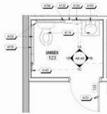
1 123 - UNISEX R.R. 3/8" = 1'-0"
