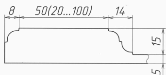
Розріз фасаду
