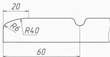
Розріз фасаду
