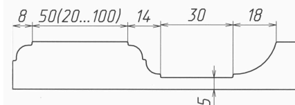
Розріз фасаду
