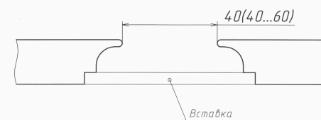
Розріз ручки
