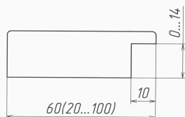
Розріз вітрини
