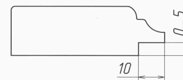
Розріз вітрини
