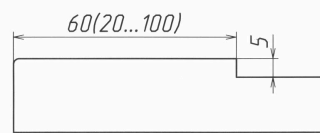
Розріз фасаду
