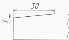
Розріз фасаду
