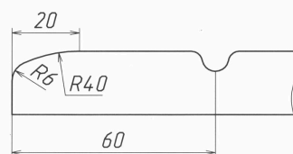
Розріз фасаду
