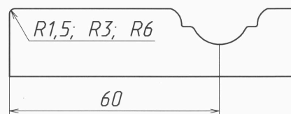
Розріз фасаду
