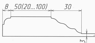
Розріз фасаду
