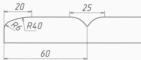
Розріз фасаду
