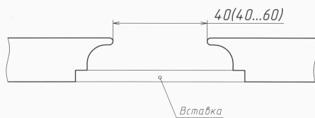
Розріз ручки
