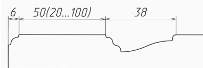
Розріз фасаду
