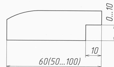
Розріз вітрини
