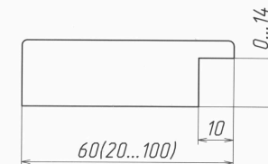
Розріз вітрини
