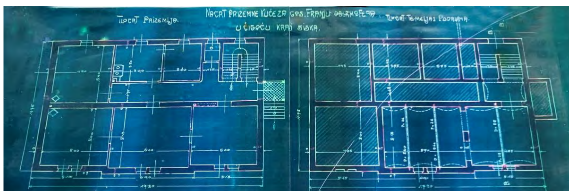
Sl. 10. Nacrt kurije Oberhofer-Hangi, 1909. god., tlocrti prizemlja i podruma (izvor: gđa. Mira Vitković)
