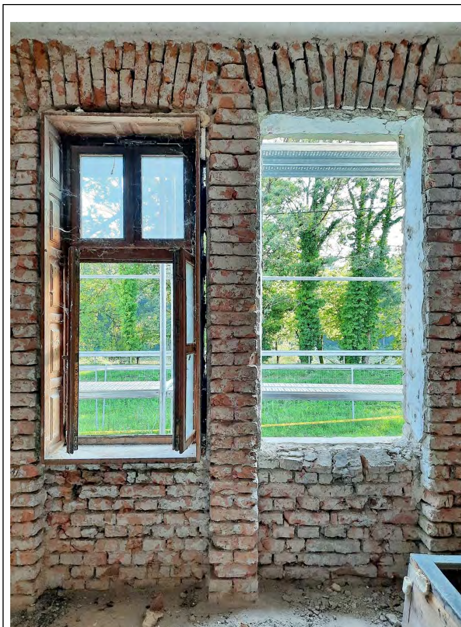
Sonda 27 – pogled iznutra, nakon uklanjanja stolarije
