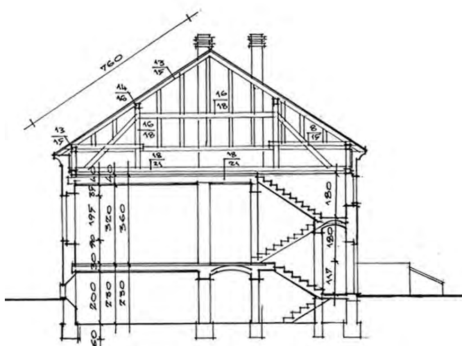
Sl. 17. Zatečeno stanje 1998. godine, presjek (izvor: N. Ljuckanov, 1998.)
