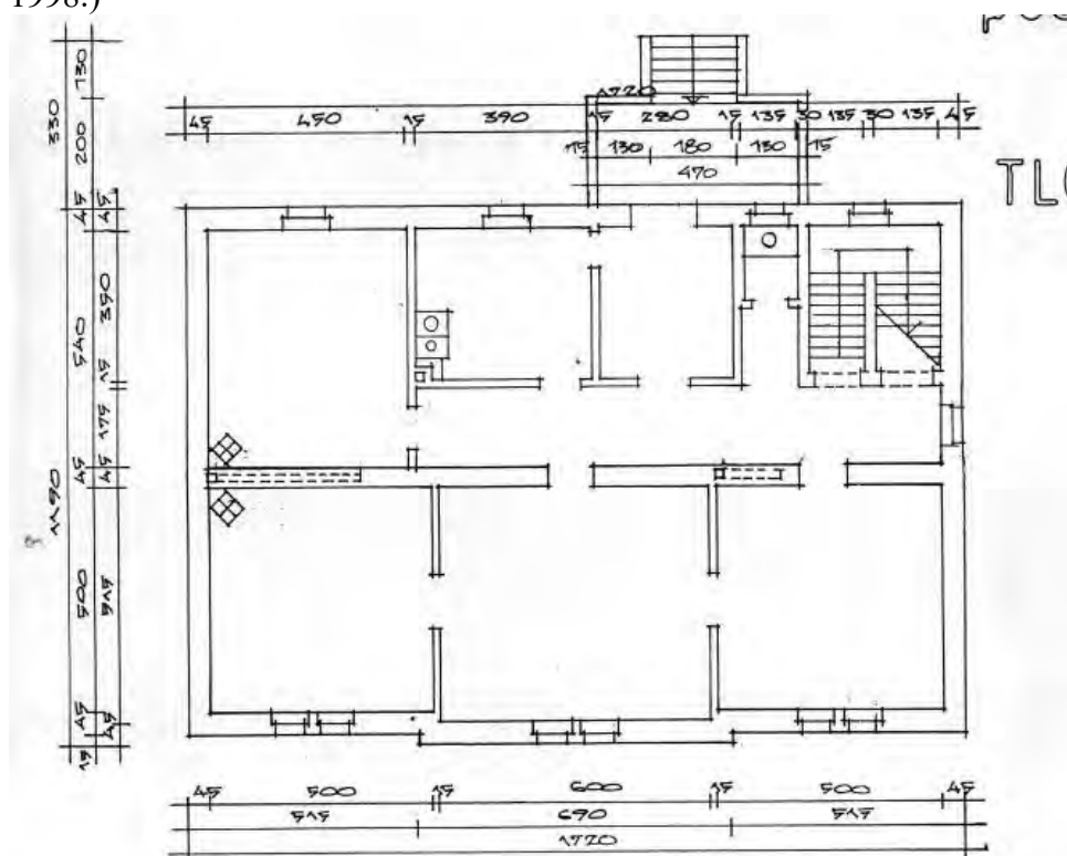
Sl. 19. Zatečeno stanje 1998. godine, tlocrt prizemlja (izvor: N. Ljuckanov, 1998.)
