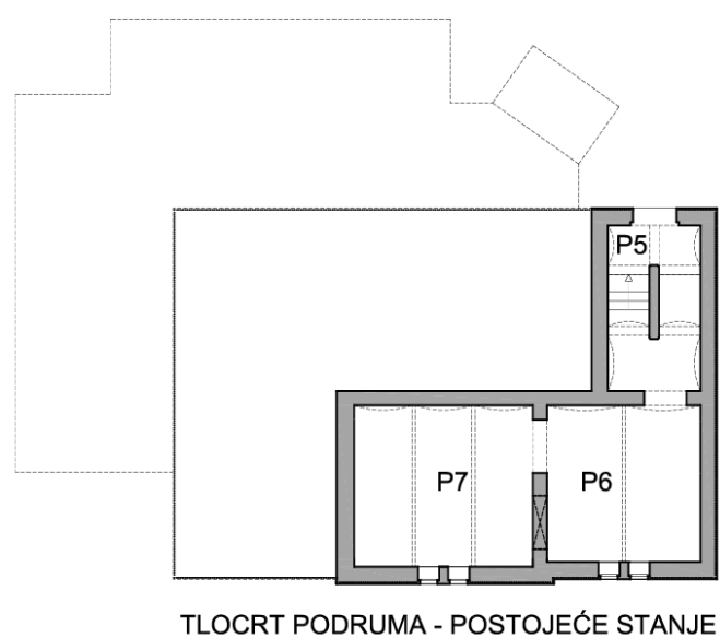
Sl. 50. Postojeće stanje – pozicija prostorija u prizemlju i podrumu
