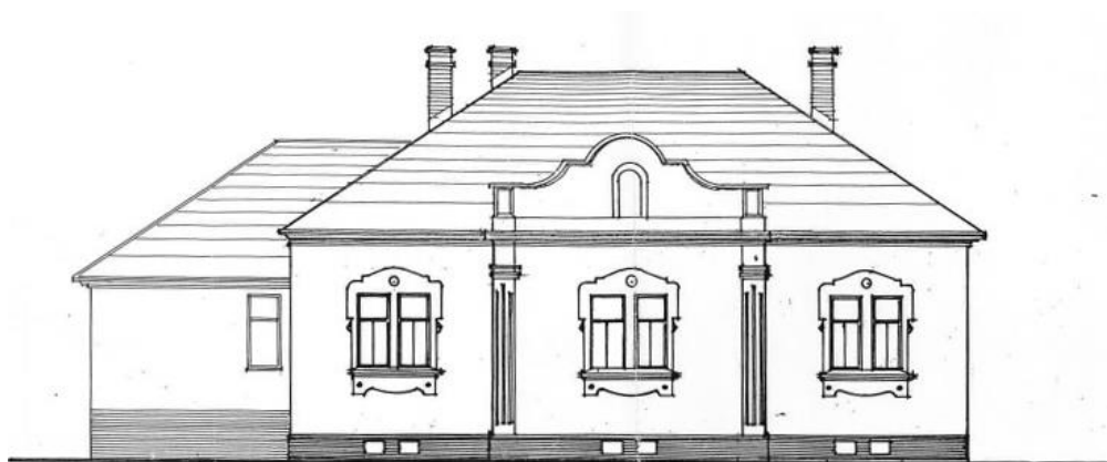
Sl. 23. Projektirano stanje 1998. godine, ulično (južno) pročelje (izvor: N. Ljuckanov, 1998.)
