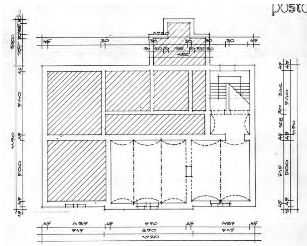
Sl. 18. Zatečeno stanje 1998. godine, tlocrt podruma (izvor: N. Ljuckanov, 1998.)
