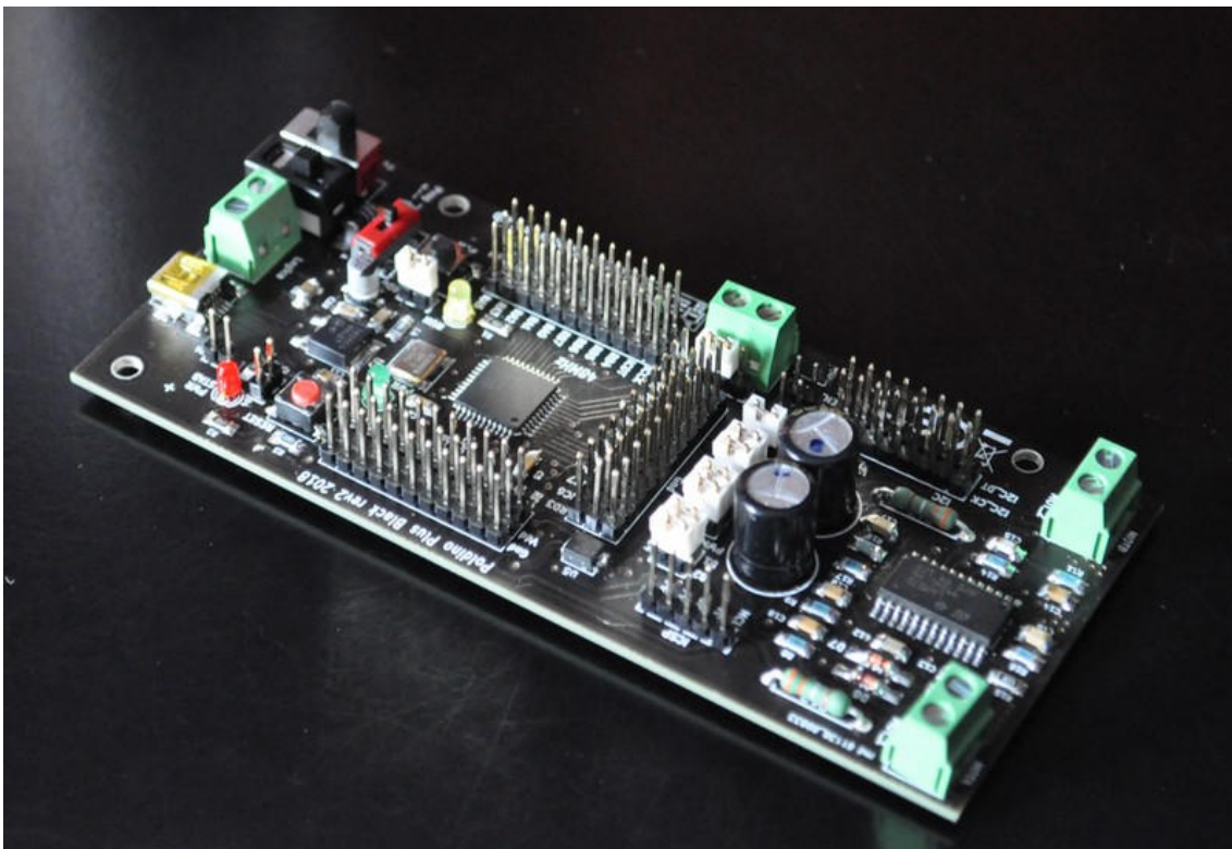
La nuova scheda PoldinoPlus Blak edition, che presenta alcune caratteristiche migliorate rispetto alla PoldinoPlus, in particolare la maggiore velocità di calcolo.
