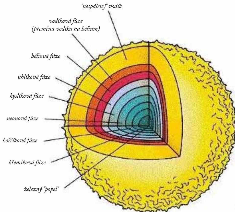
Ideální řez hvězdou, která ve svém žhavém nitru přeměňuje lehké prvky na těžší.
