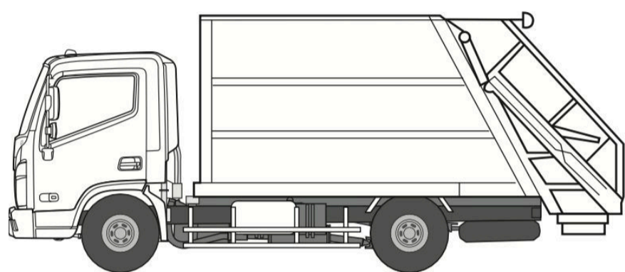
Мусоровоз с загрузкой заднего типа с прессом
