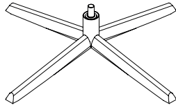
S09 Standard m/treverk / S09 Høy m/treverk Svartlakkert eller børstet stål senter søyle
