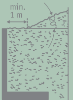
B | Böschung Geländenei- gung 20^\circ , Ver- kehrslast bis p = 5 \text{ kN/m}^2 , 1 m Abstand
