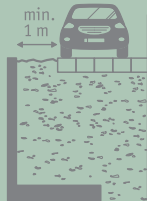
A | Verkehrs- last bis p = 5 \text{ kN/m}^2 ohne Anprall- lasten, 1 m Abstand
