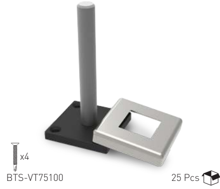
AK-5234 Base Flange for 40x40 Baluster Post 40x40 Dikme İçin Yer Bağlantı Flanşı
