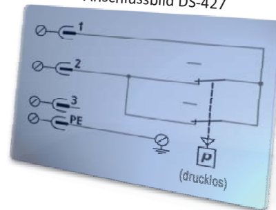
Anschlussbild DS-427
