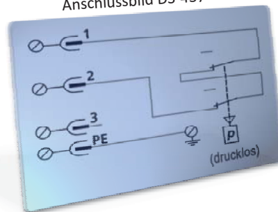
Anschlussbild DS-437
