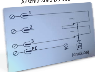
Anschlussbild DS-432
