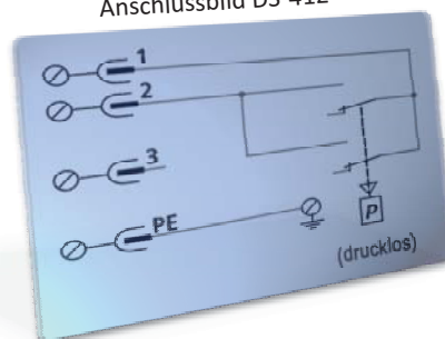
Anschlussbild DS-412
