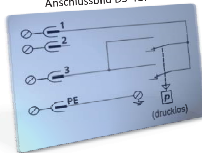
Anschlussbild DS-417
