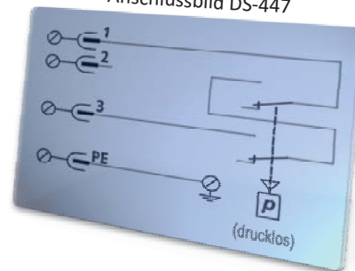
Anschlussbild DS-447
