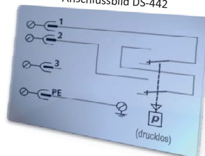
Anschlussbild DS-442
