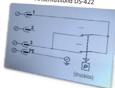
Anschlussbild DS-422
