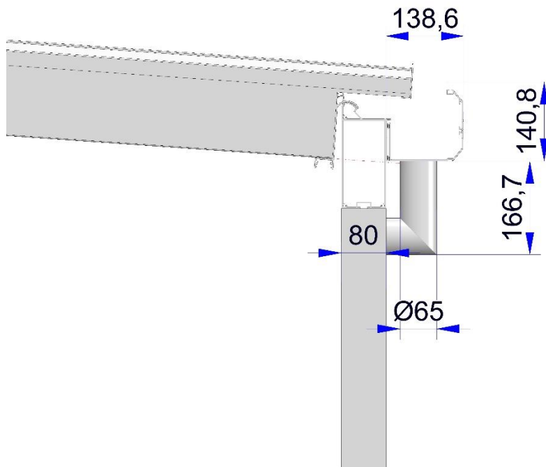
Bild 4: Schnitt Traufe
