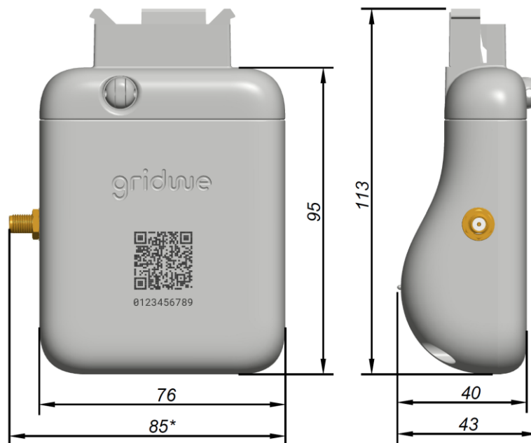
Рисунок 1 - Габаритні розміри модему
