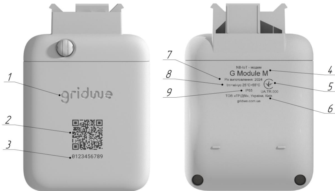
Рисунок 3 - Зразок маркування
