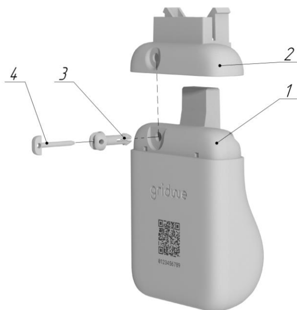
Рисунок 2 - Конструкція модему
