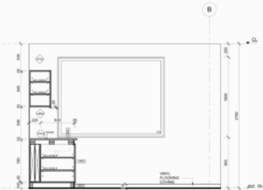
3 CRECHE 02 ELEVATION B 1:20
