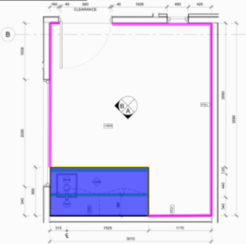
1 CRECHE 02 PLAN 1:20
